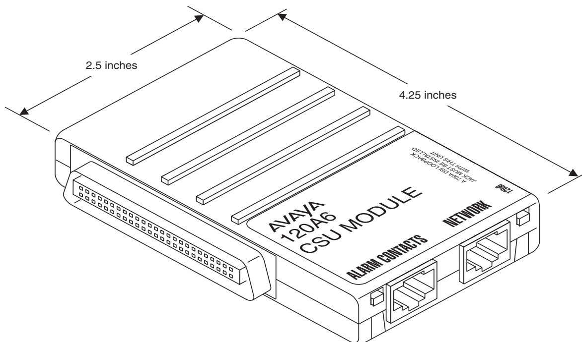
Figure 59: 120A CSU
